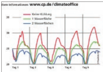
Entwicklung der Raumtemperatur im Büro, wenn Wasserflächen installiert werden. Messungen aus 2016 im Fraunhofer IBP
