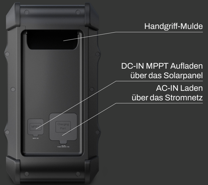
RÜCKANSICHT
